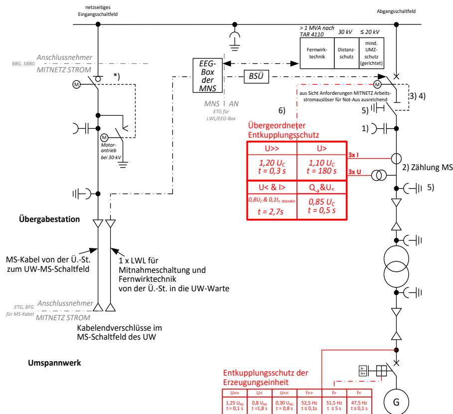
Abb. 24: (ehemals D3a): \leq 20\text{-kV} und 30\text{-kV} UW-MS-Sammelschienenanschluss einer Erzeugungsanlage
