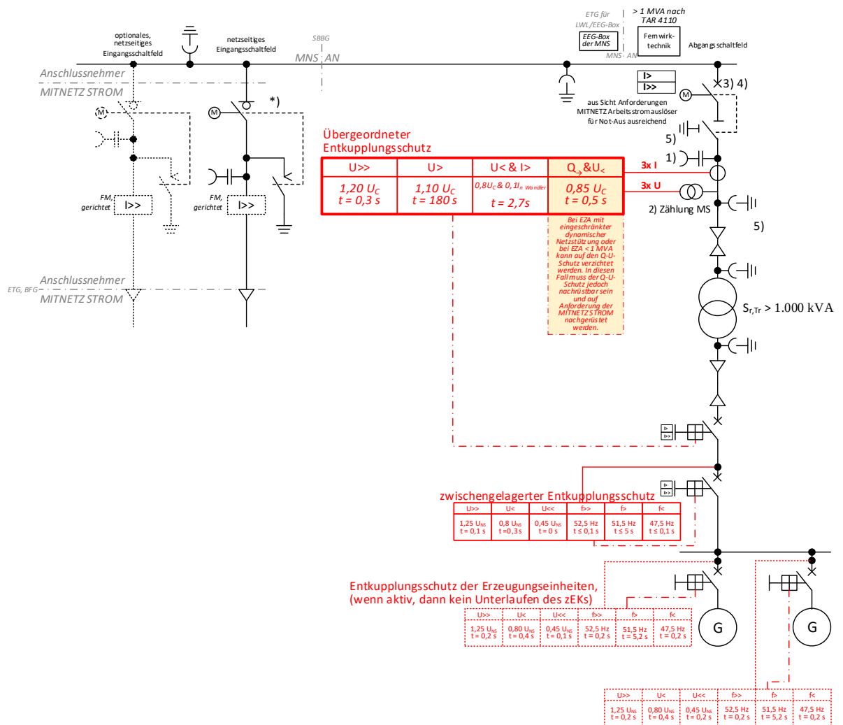
Abb. 28: (ehemals D4d): ≤ 20-kV- Anbindung einer Erzeugungsanlage &gt; 1 MVA
