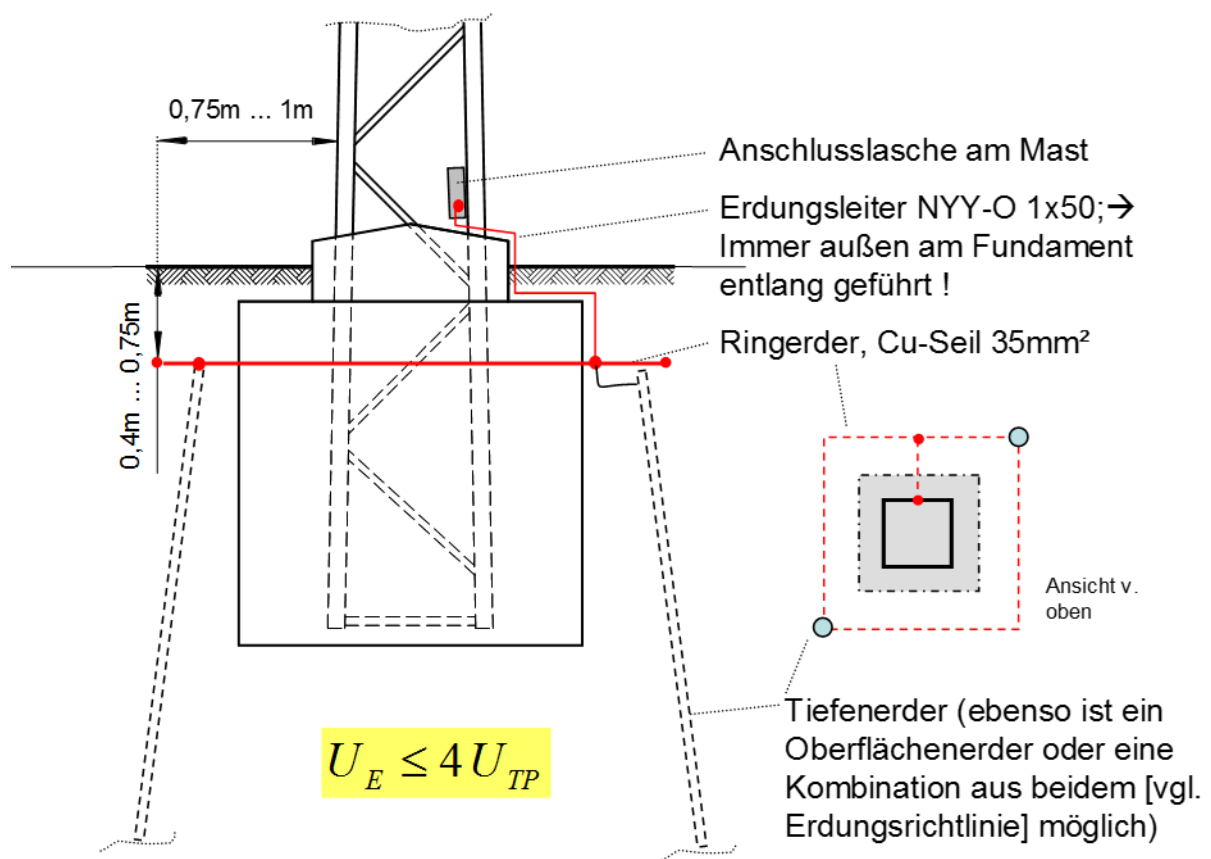
Abb. 6: Standard-MS-Mast-Erdsanlage
